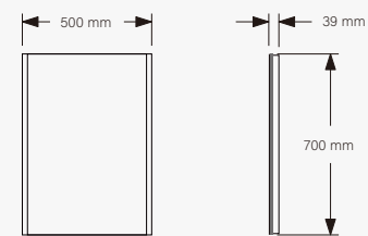
Vorderansicht
