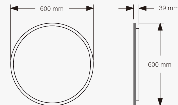
Vorderansicht
