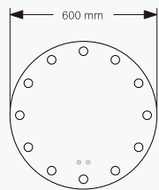
Vorderansicht
