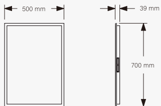
Vorderansicht
